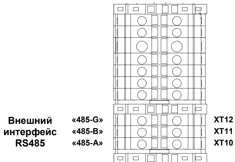
Рисунок Л.3 - Схема подключения цепей внешнего интерфейса (панель А19)
