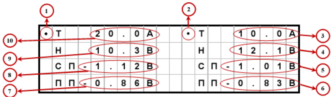
Рисунок Ж.1 – Основной информационный экран блока БКУ-01
