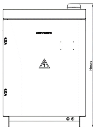
Рисунок А.2 Габаритные и установочные размеры преобразователей исполнения ПН-ОПЕ-М11-...-А.2-GPRS.EM1
