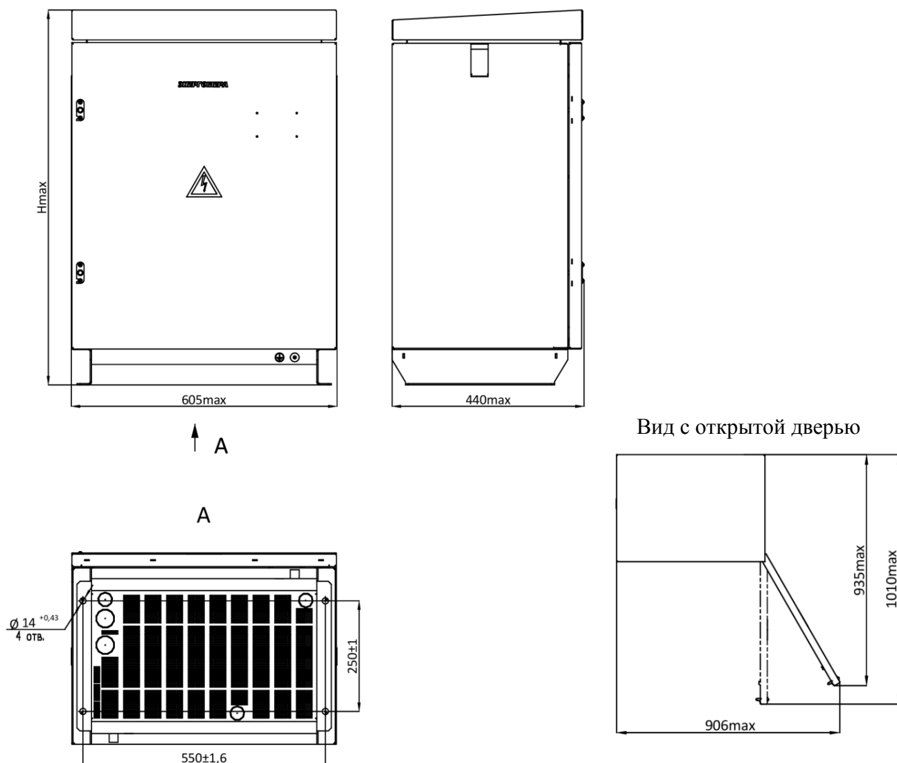
Рисунок А.1 Габаритные и установочные размеры преобразователей исполнения ПН-ОПЕ-М11-...-А.2-485
