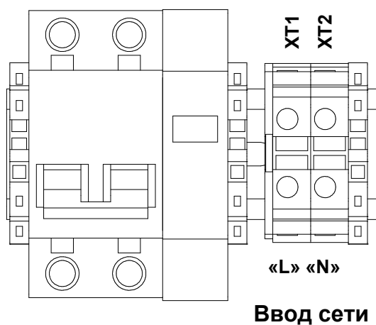
Рисунок Л.1 - Схема подключения сети питания (панель сетевая А1)
