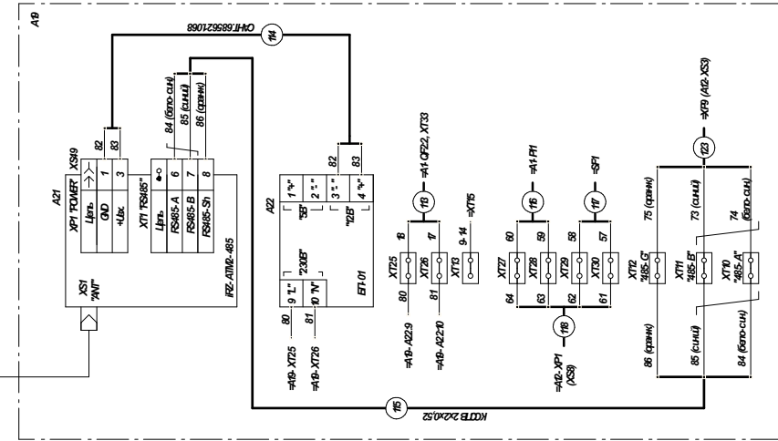
Рис.5 (продолжение А2) Для станций СНГ.А53241002-48...95 Отличие см. рис.1,2
