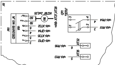
Рис.3 (продолжение Р1) Для станций СНГ.А53241002-32...47...80...95 Отличие см. рис.1,2
