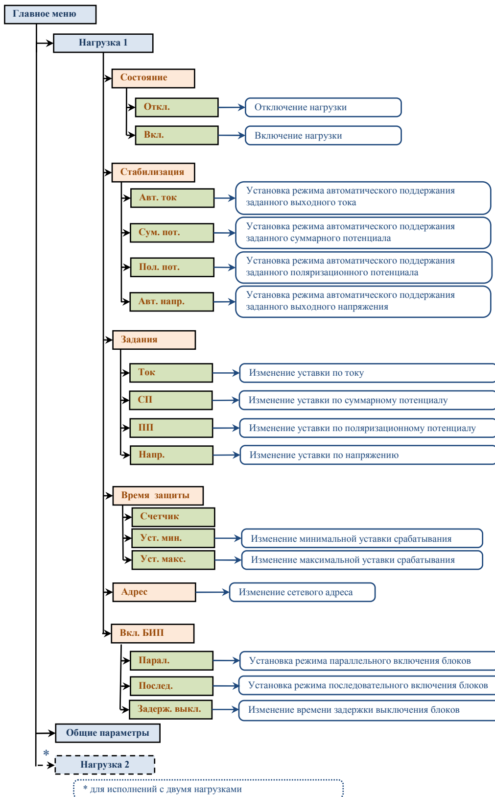
Рисунок И.1 – Структура меню блока БКУ-01 «Нагрузка»
