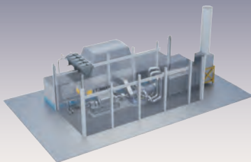
Стационарная газовая энергетическая турбина ГТ-009М(МЭ) собственной разработки
