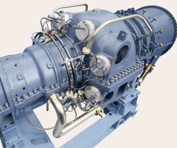
Стационарная газовая энергетическая турбина ГТ-009М(МЭ) собственной разработки
