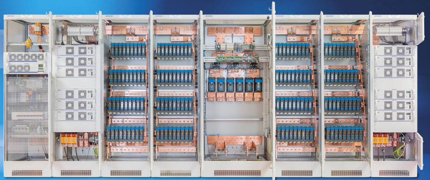
Modulares Stromversorgungssystem für einen Telekommunikationsknotenpunkt Modular power supply system for a telecommunications hub
