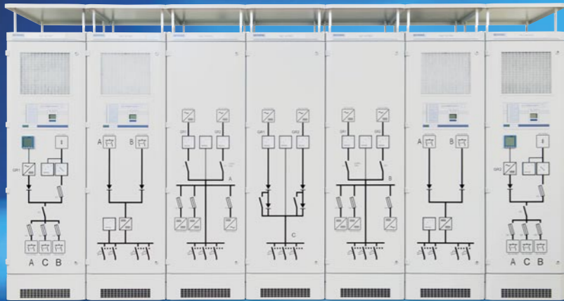
Eigenbedarfsstromversorgung eines Wasserkraftwerkes Internal power supply of a hydrofacility
