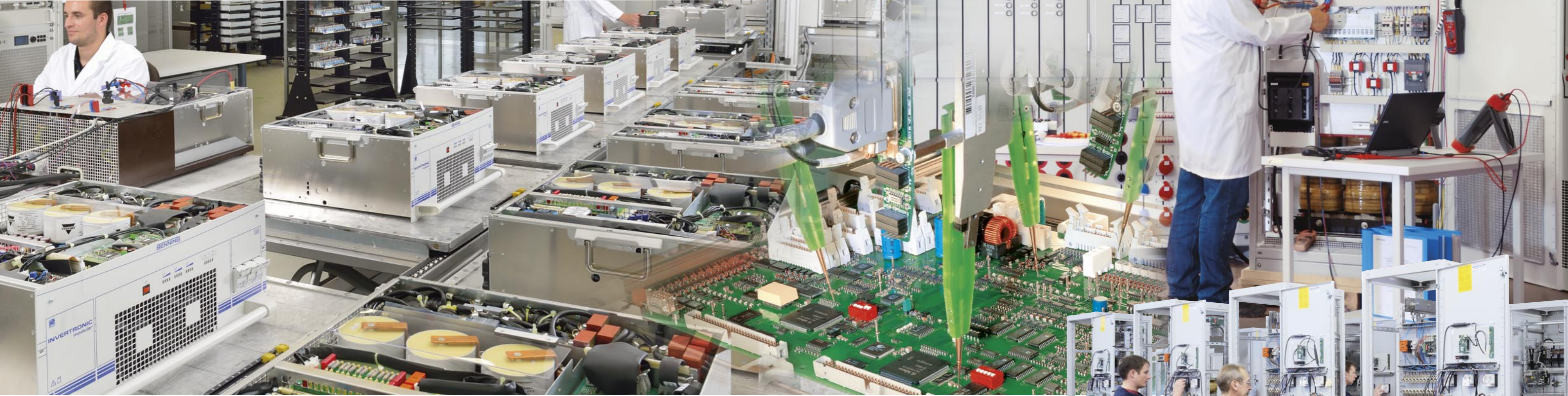
Montage und Prüffeld von Wechselrichtereinschüben Invertör modülü montaj ve test bölümü
